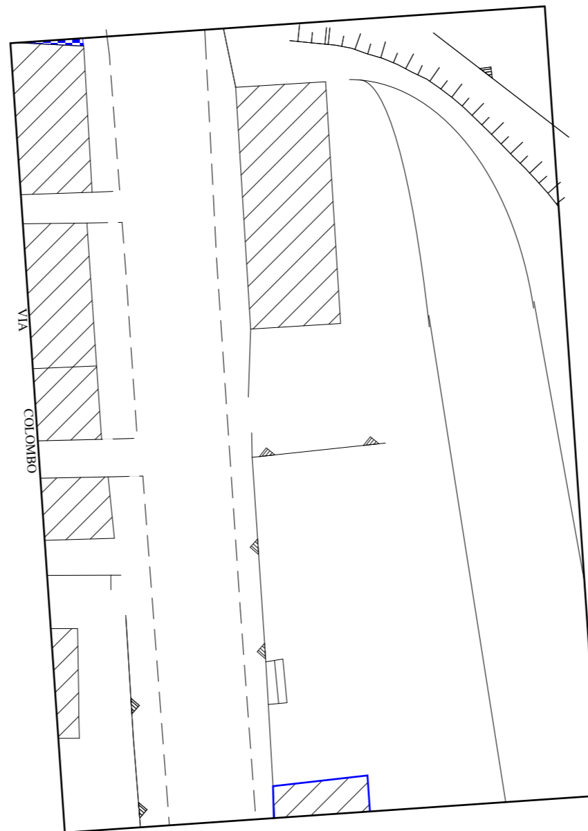
STRALCIO AEROFOTOGRAMMETRICO 1:500
